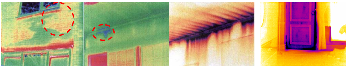
建筑物外墙 大面积受潮
