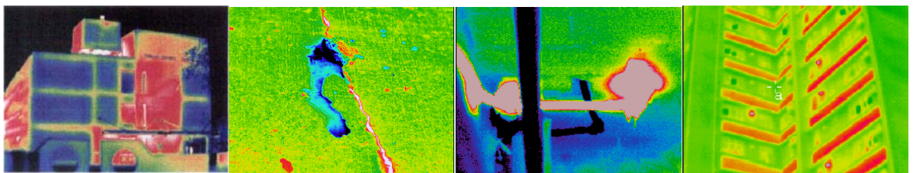
建筑节能检测 热桥
