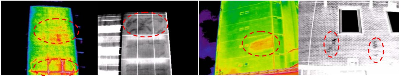
结构缺陷 裂缝
